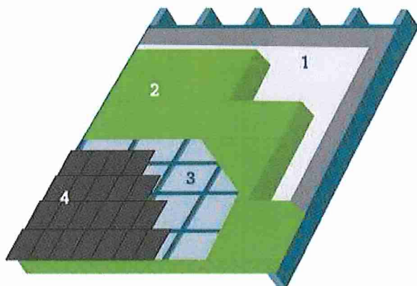
1. Dampschermelement | 2. Isolatie | 3. Onderdak | 4. Dakbedekking
